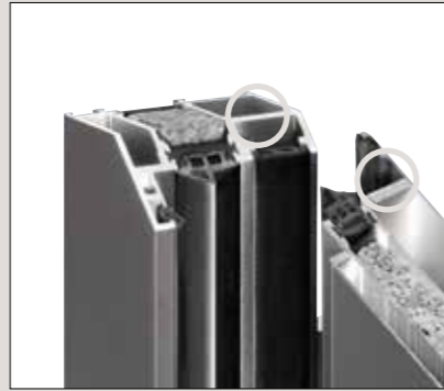
Wandungsstärke bis 3 mm bietet einen sicheren Halt für Schloss und Bandbolzen
