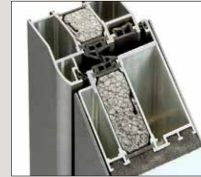
3 Dichtungsebenen garantieren optimalen Schutz gegen Wärmeverlust durch Zugluft
